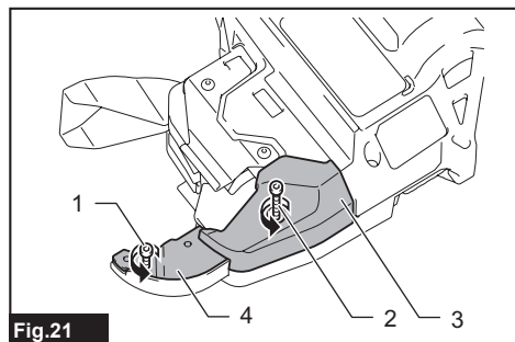
Fig.21 ► 1. Boulon A 2. Boulon B 3. Couvercle de la plaque de contact 4. Guide-fil B équipé standard (argenté)
