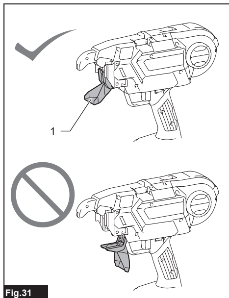
► 1. Guide-boucle
