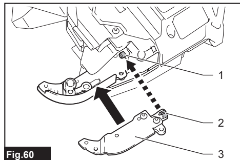
Fig.60 ► 1. Pipe 2. Groove 3. Wire guide B
