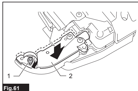
Fig.61 ► 1. Bolt A 2. Wire guide B
