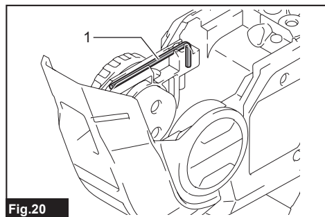
Fig.20 ► 1. Clé hexagonale
